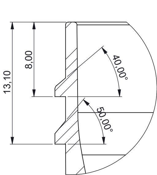
DETALHE C ESCALA 4 : 1
