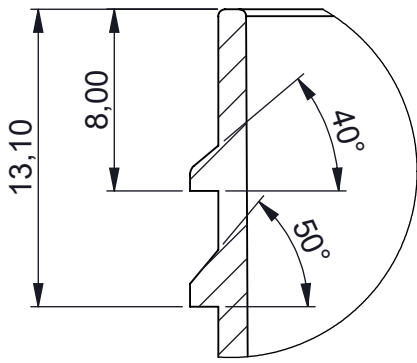
DETALHE C ESCALA 3 : 1
